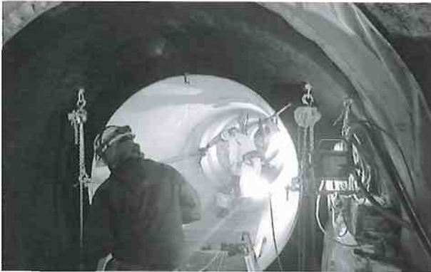
取水トンネル内に導水管（直径1.8m）を敷設
