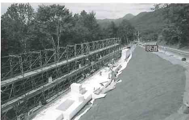
急峻な山岳道路のため、軽量盛土材にて施工しています。現場では、全面通行止めが困難なため、昼夜2交代で作業しています。
